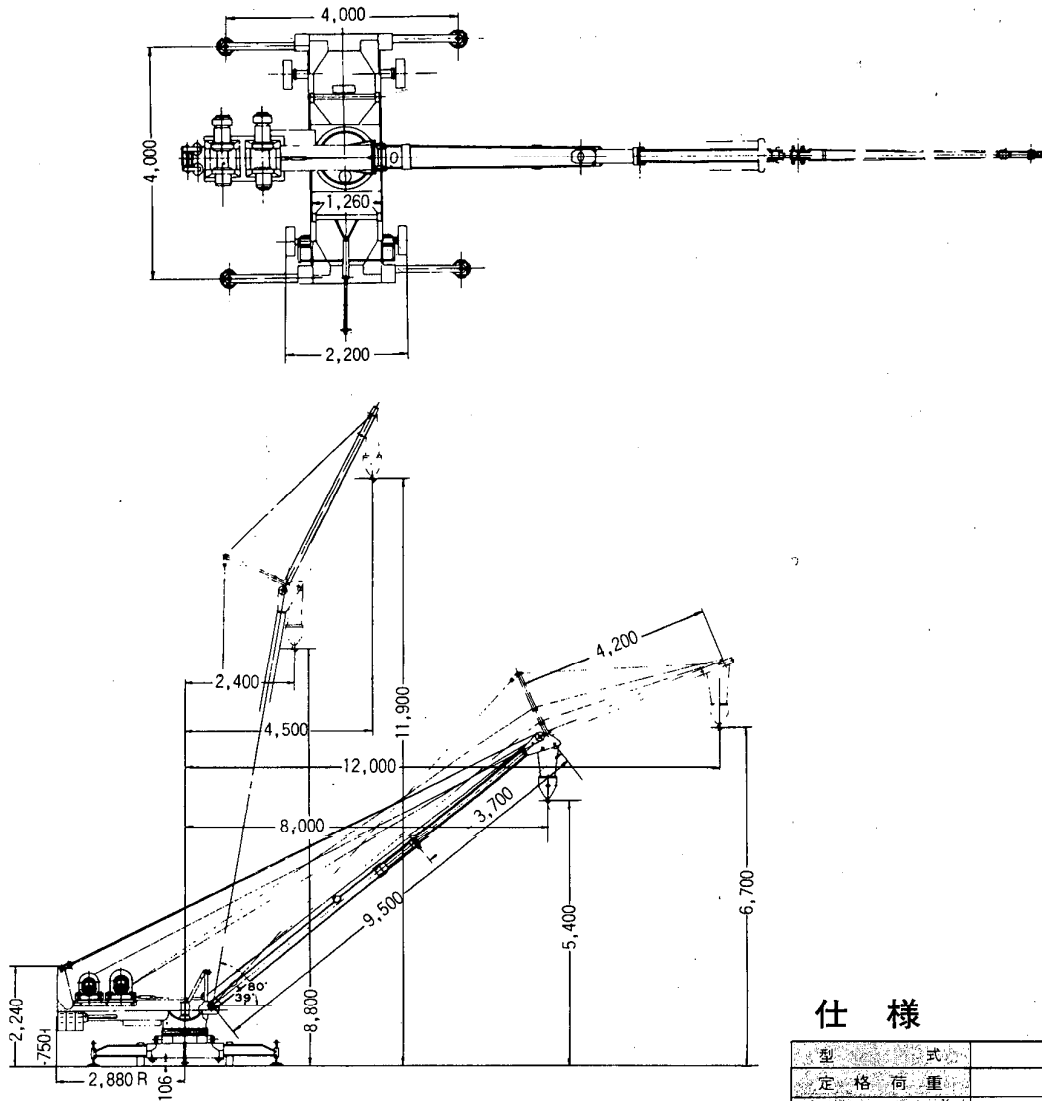
主要寸法図 単位：mm
