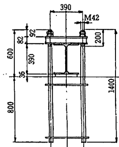
アンカーボルト図
