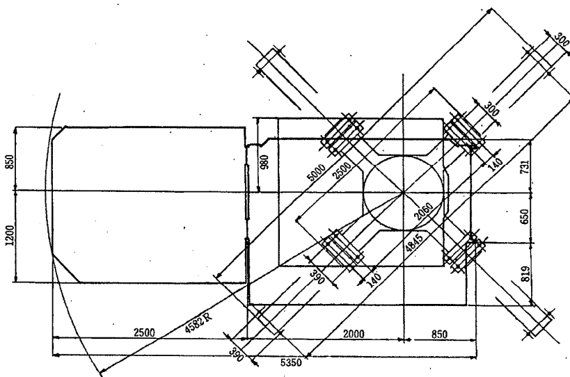
平面寸法図
