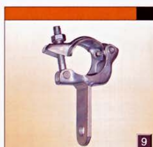
●朝顔クランプ舌付 60ミリ 1個 0.5kg 70ミリ 1個 0.5kg
